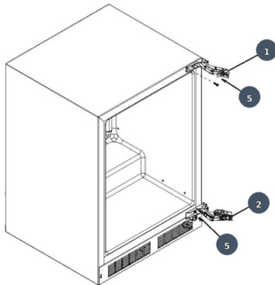
Right Hand Door Hinging
