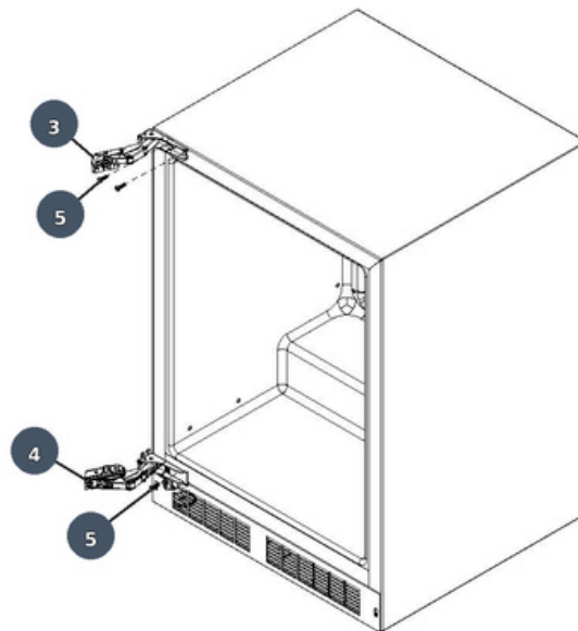
Left Hand Door Hinging
